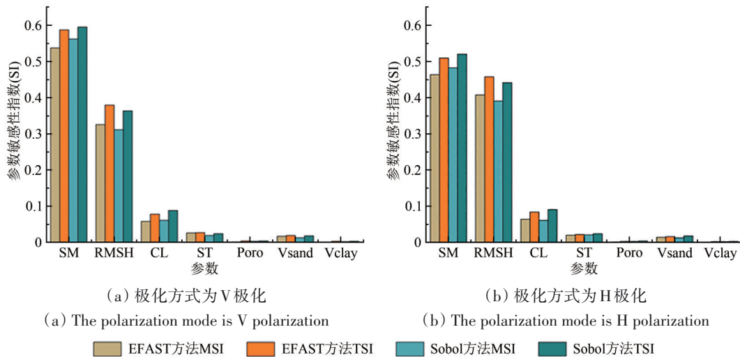
图1 基于EFAST和Sobol'算法的参数定量敏感性分析(根据(Ma等,2017b)有改动)
